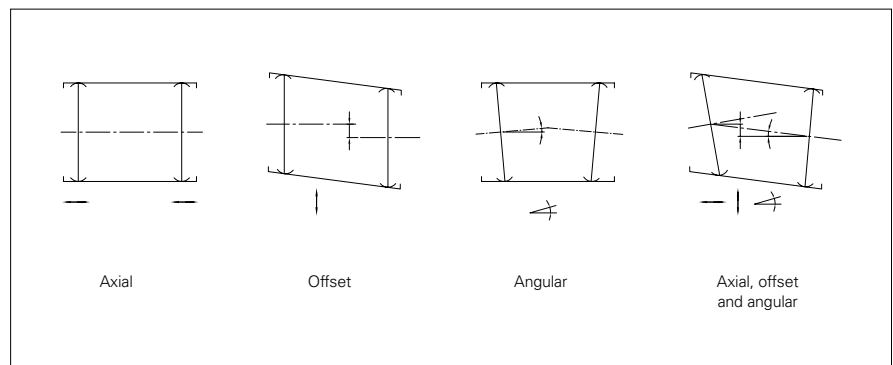
Fig. n.º 3. Shaft misalignment.
