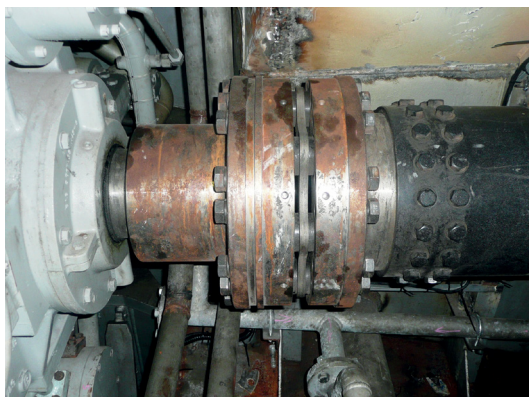
LAMIDISC coupling DOM-410- 8
